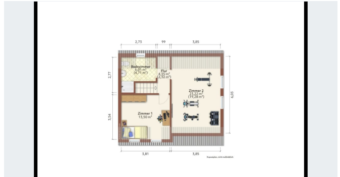
Grundriss DG0
